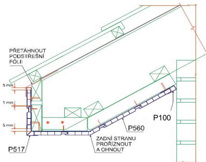
Obrázek 3: Podbití krovu se šikmou spodní částí, obkladové lamely příčně – kolmo na fasádu
